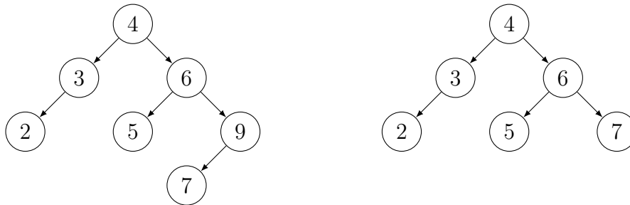
22. ábra. A bal oldali bináris keresőfa legnagyobb kulcsú csúcsát eltávolítva a jobb oldalit kapjuk: Az eredeti fa jobb szélső csúcsát kivesszük, és a saját bal részfájával helyettesítjük. Vegyük észre, hogy az eredeti fából a 9 kulcsú csúcs törlése is ugyanazt a fát eredményezi.
