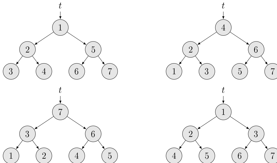
16. ábra. Bal felső sarokban preorder, jobb felsőben inorder, bal alsóban postorder, jobb alsóban szintenkénti bejárása látható a t bináris fának.
