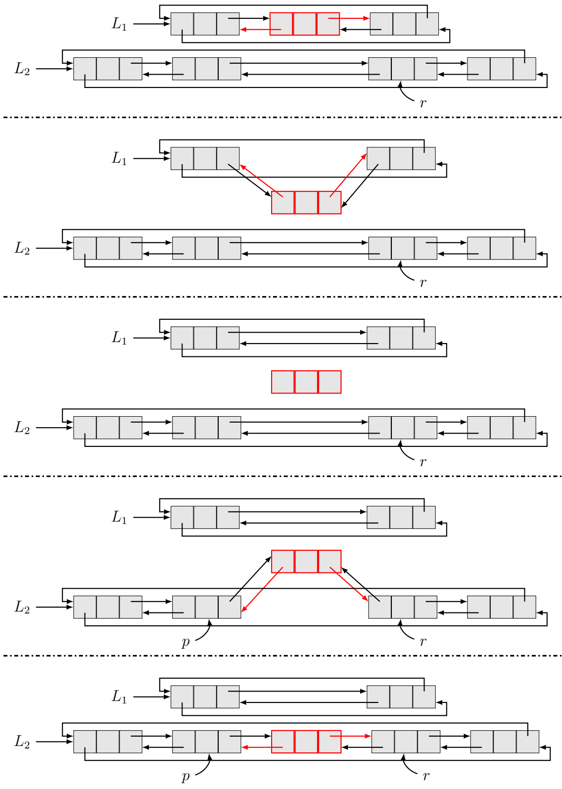
7. ábra. Az unlink(q) és a precede(q, r) metódus szemléltetése. A piros listaelemre ( *q ) hívjuk meg a beszúrás, és ( *r )-től balra kerül beszúrásra L_2 listába.
