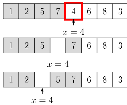
1. ábra. A beszúró rendezés szemléltetése.
