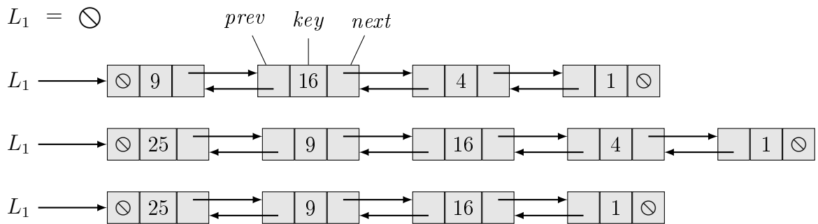
5. ábra. Az L_1 mutató egyszerű kétirányú listákat (S2L) azonosít egy képzületbeli program futásának különböző szakaszaiban. Az első sorban a listát üresre inicializáló értékadás látható.
