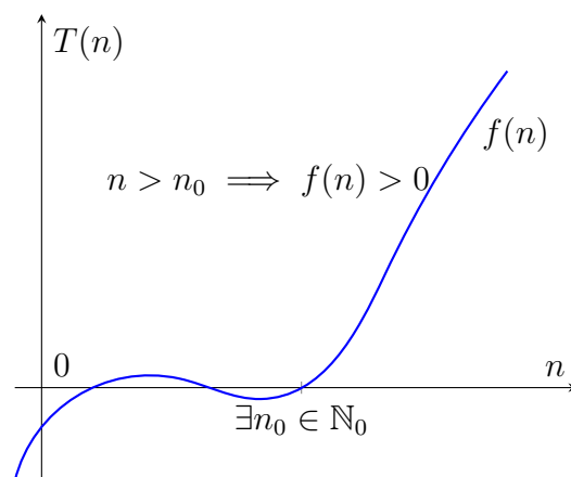
8. ábra. Aszimptotikusan pozitív (AP) függvény
