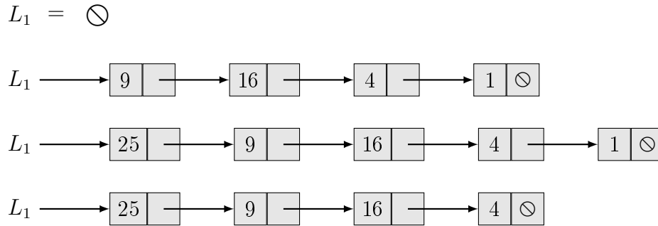
3. ábra. Az L_1 mutató egyszerű egyirányú listákat azonosít egy képzeletbeli program futásának különböző szakaszaiban. Az első sorban a lista, üres lista állapotában látható.
